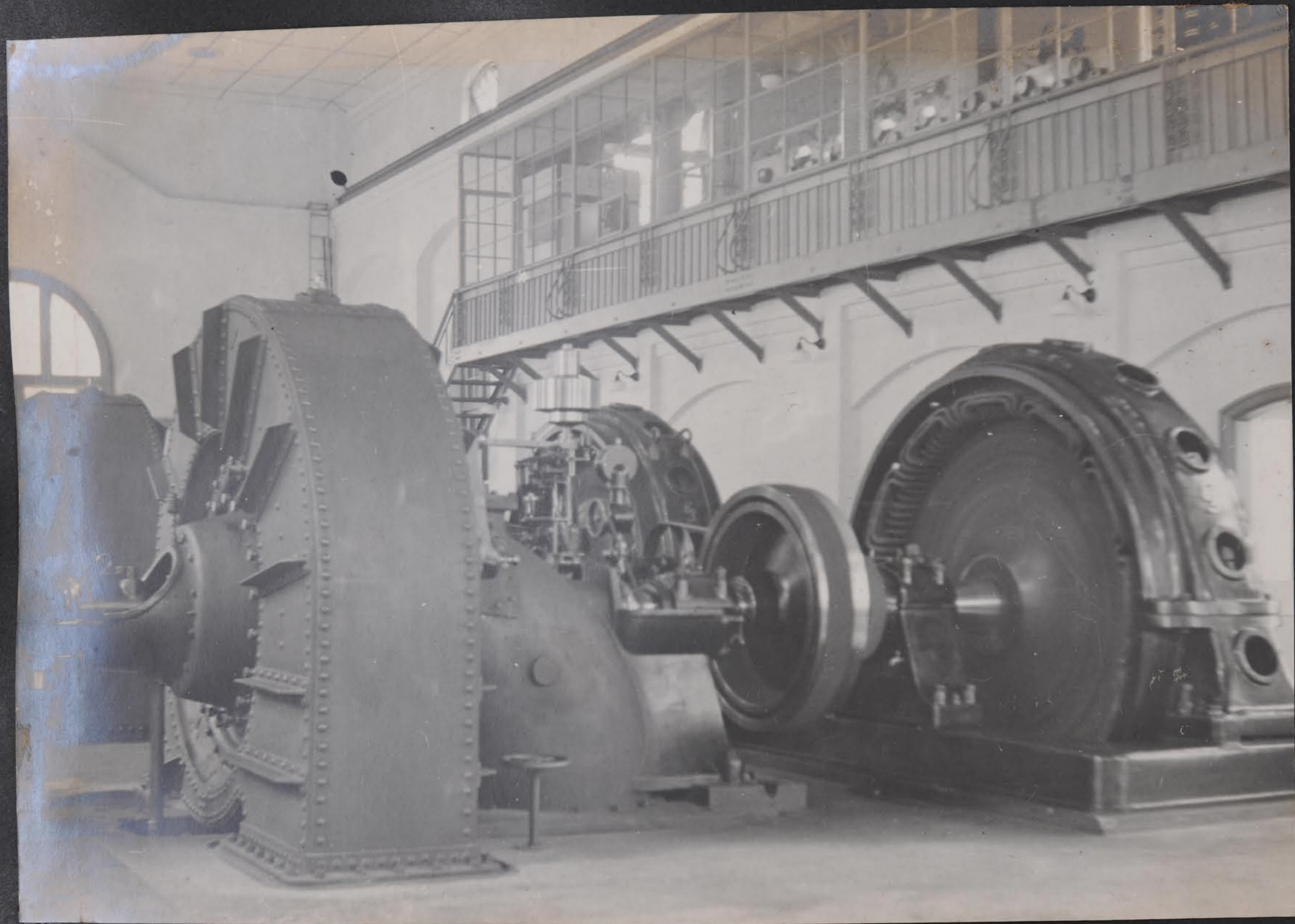
吉野第一發電所發電機
