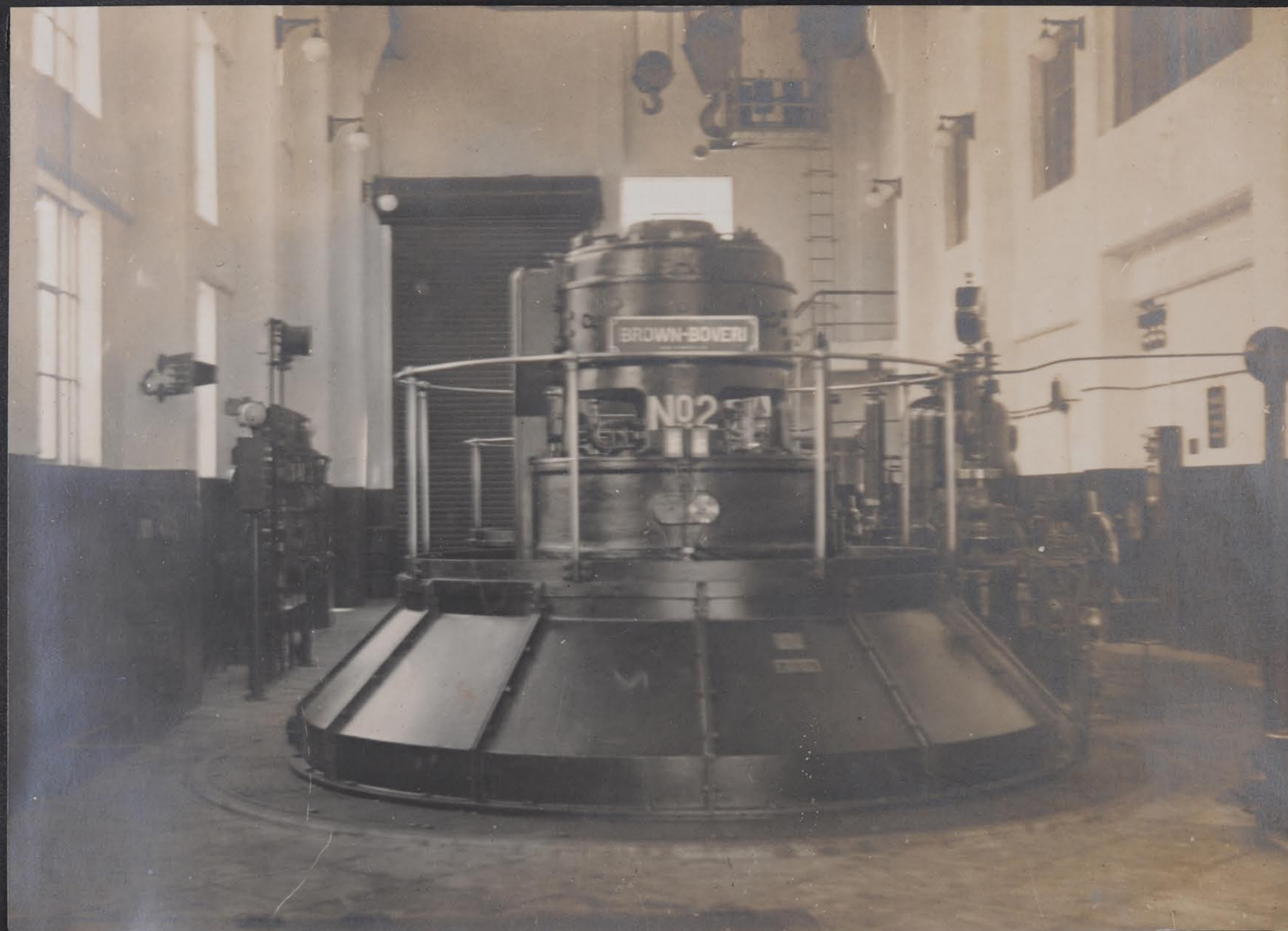
鳥越發電所發電機
