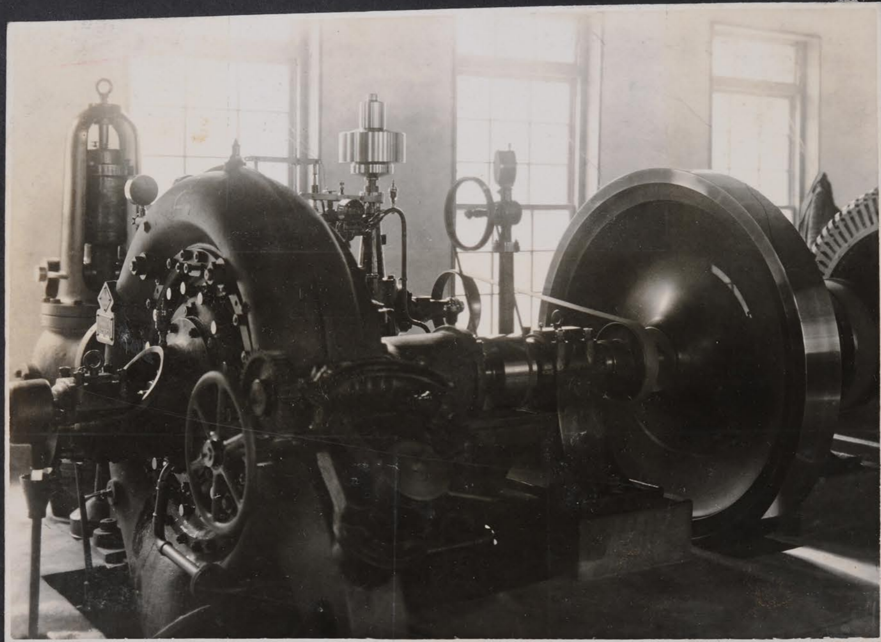
辰巳發電所發電機
